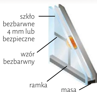
Zespolony pakiet szklany dwukomorowy FLOAT/ SZKŁO PIASKOWANE + JEWEL/ REFLEX
