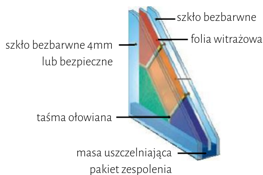
Zespoleony pakiet szklany dwukomorowy FLOAT/ FOLIA WITRAŻOWA + OŁÓW/ FLOAT
