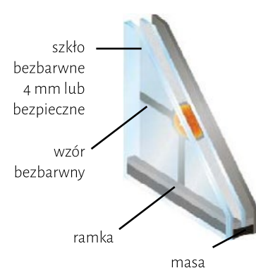
Zespolony pakiet szklany dwukomorowy FLOAT/ SZKŁO PIASKOWANE + JEWEL/ REFLEX
