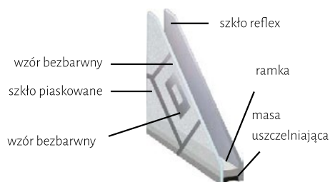
Zespolony pakiet szklany jednokomorowy SZKŁO PIASKOWANE/ REFLEX
