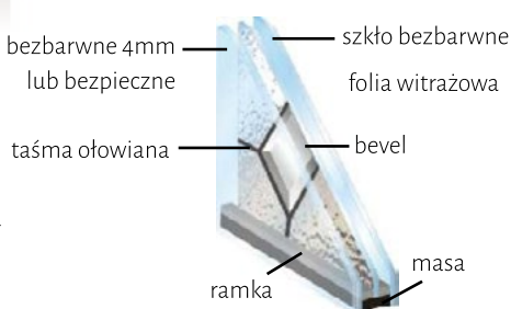
Zespolony pakiet szklany dwukomorowy FLOAT/ WITRAŻ + BEVEL/ FLOAT
