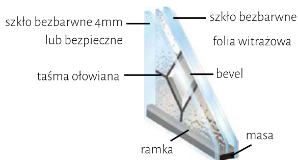
Zespoleony pakiet szklany dwukomorowy FLOAT/ WITRAŻ + BEVEL/ FLOAT
