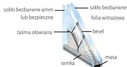
Zespolony pakiet szklany dwukomorowy FLOAT/ WITRAŻ + BEVEL/ FLOAT
