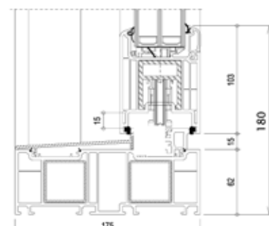
Przekrój pionowy dolny
