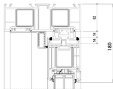
Przekrój pionowy górny
