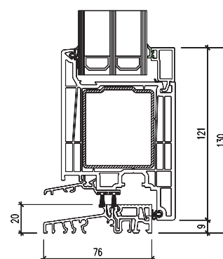
VP 80 DECEUNINCK
